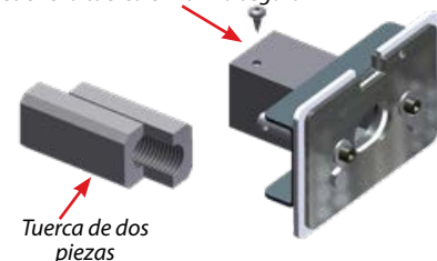
El bloqueo de metal de desplazamiento retiene la tuerca en forma segura
