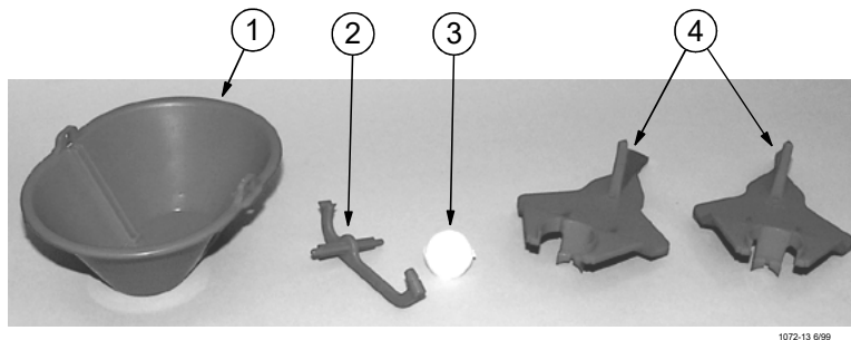
Figure 1. Mini Drinker Components
